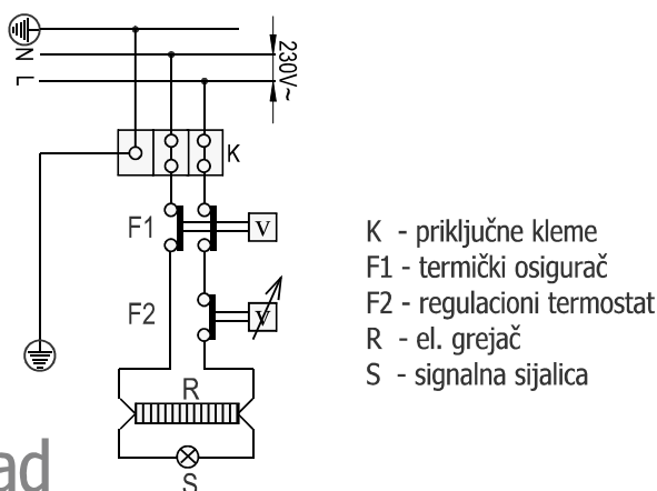
Elektro šema
